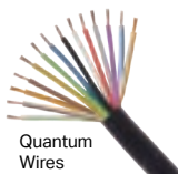
Quantum Wires
